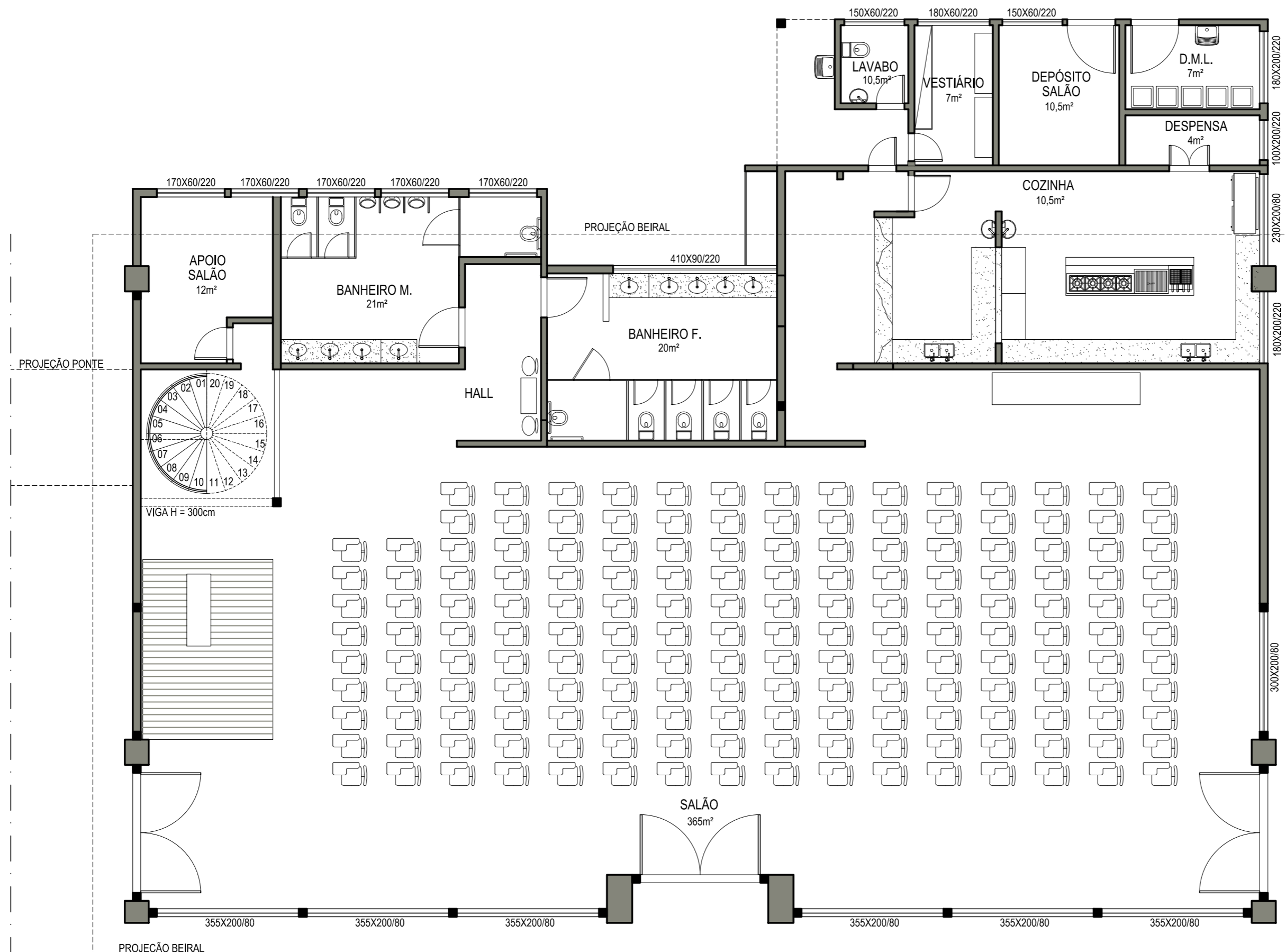
LAYOUT SALÃO 1º PAVTO. ESCALA 1/100
